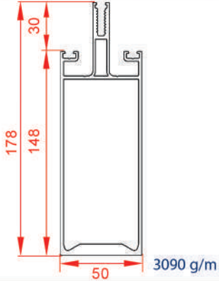
لامل عمودی ۱۷۸
