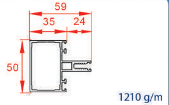
لامل افقی ۵۹
