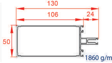
لامل افقی ۱۳۰
