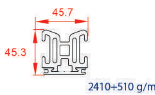
لقمه کشویی دو تکه
