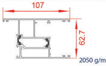
لنگه سیستم لیفت
