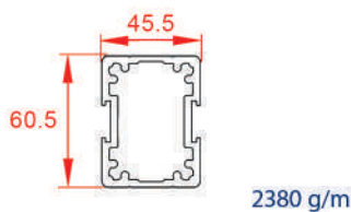
لقمه مولیون ۱۱۰
