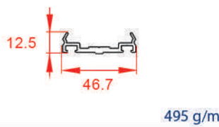
زهوار درپوش
