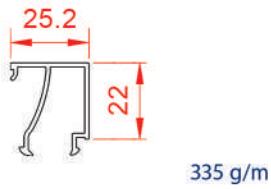
زهوار دو جداره
