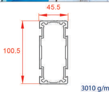
لقمه مولیون ۱۵۵
