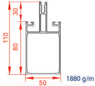
لامل عمودی ۱۱۰
