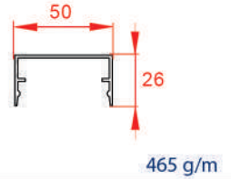
درپوش ۲۶
