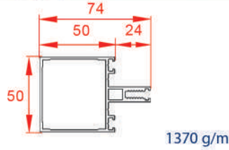
لامل افقی ۷۴
