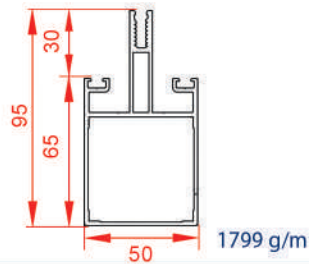
لامل عمودی ۹۵
