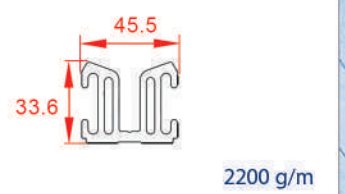
لقمه فیکس
