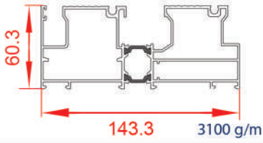
فریم سیستم لیفت
