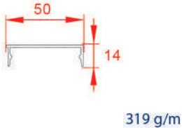
درپوش ۱۴
