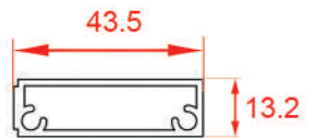
پروفیل وسط چهار لنگه
