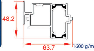
پروفیل وسط چهار لنگه
