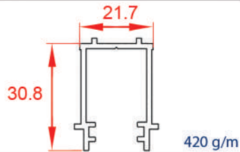
اسپیسر یراق UPVC
