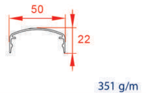
درپوش قوس دار ۲۲
