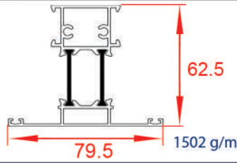
پروفیل سپری
