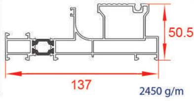
فریم مونوریل
