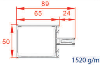
لامل افقی ۸۹
