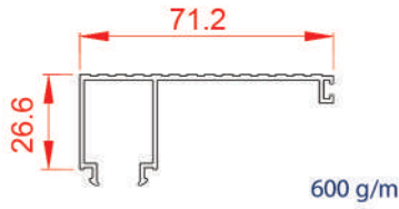
درپوش مونوریل
