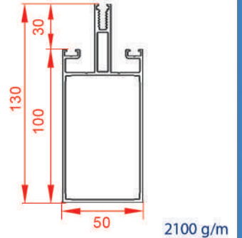
لامل عمودی ۱۳۰
