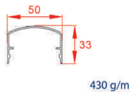
درپوش قوس دار ۳۳
