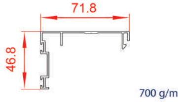
درپوش لنگه سیستم لیفت
