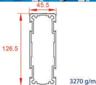
لقمه مولیون ۱۷۸
