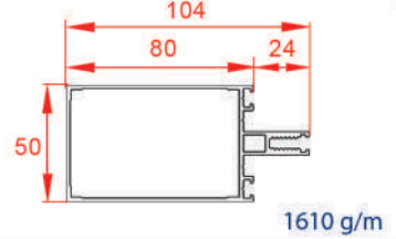
لامل افقی ۱۰۴
