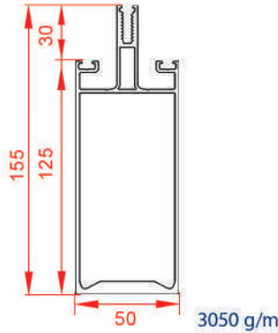
لامل عمودی ۱۵۵
